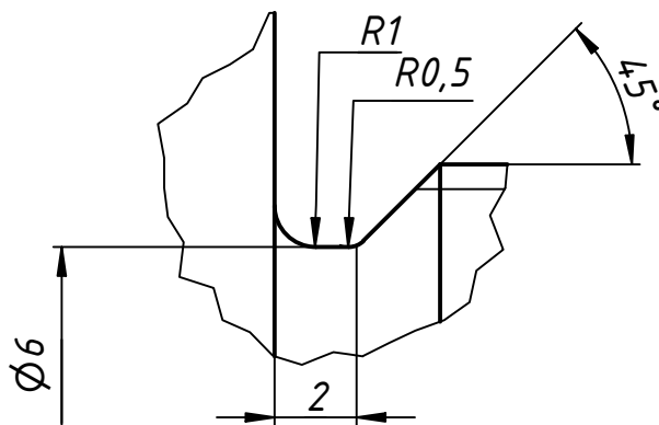
A (5 : 1)
