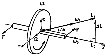
Фиг. 20.2. Гироскоп.
