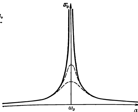
Ф и г. 25.5. Резонансная кривая, отражающая разнообразные виды трения.
