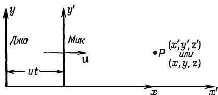
Фиг. 15.1. Две системы координат, находящиеся в равномерном относительном движении вдоль оси x .
