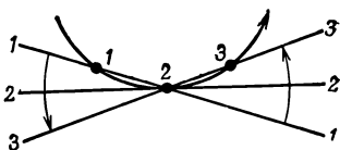
Фиг. 19.4. Три последовательных положения движущейся по радиусу точки вращающегося стола.
