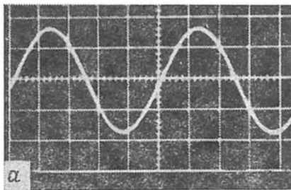
Фиг. 5.2. Две осциллограммы, снятые с экрана осциллографа. а—при осциллографе, подключенном к одному осциллятору; б—при осциллографе, подключенном к осциллятору, период колебаний которого в десять раз меньше первого.
