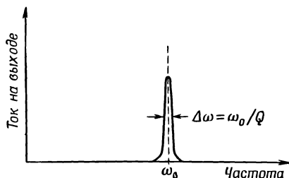
Ф и г. 23.10. Кривая отклика на частоту для резонансной полости.
