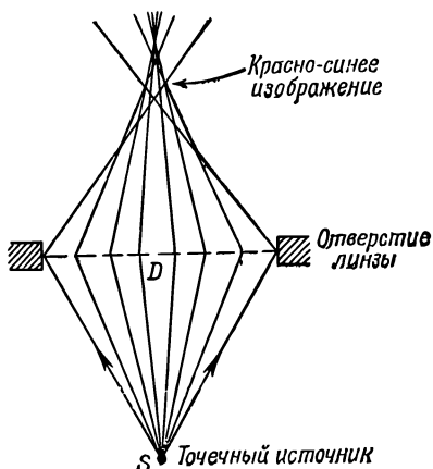
Ф и г. 29.9. Сферическая aberrация линзы.
