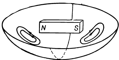
Фиг. 16.9. Магнитная палочка отталкивается вихревыми токами и висит над чашей из сверхпроводника.
