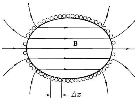
Ф и г. 29.4. Внутри эллипсоидальной катушки, ток которой на любом интервале оси \Delta x одинаков, возникает однородное поле.
