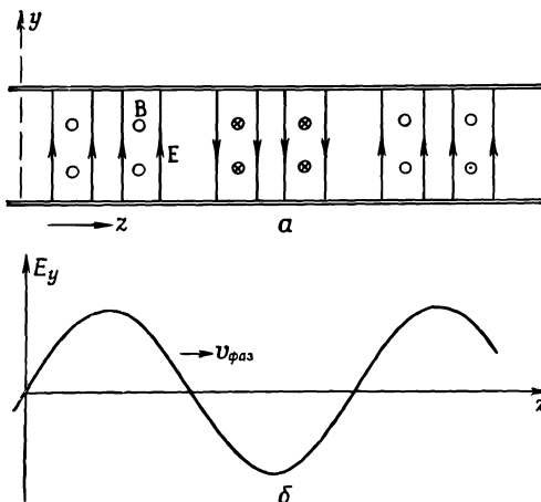
Ф и г. 24.5. Зависимость поля в волноводе от z .
