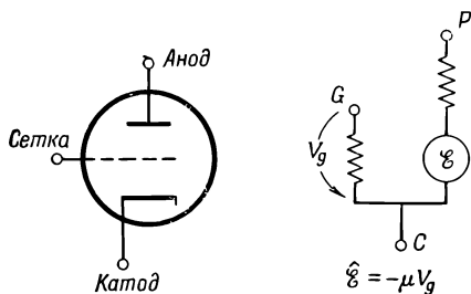
Ф и г. 22.28 Низкочастотная эквивалентная схема вакуумного триода.
