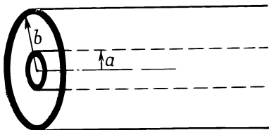
Фиг. 24.1. Коаксиальная передающая линия.
