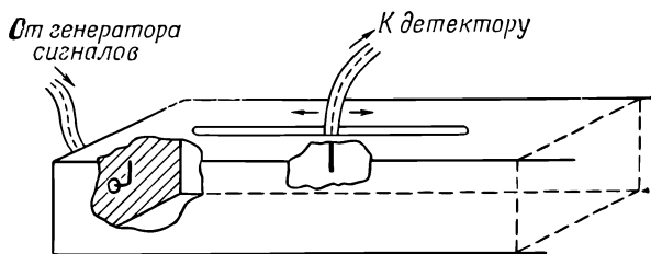
Фиг. 24.8. Волновод с входным штырем и пробником.
