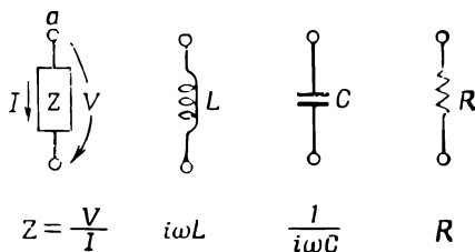
Ф и г. 22.4. Идеальные сосредоточенные элементы цепи (пассивные).
