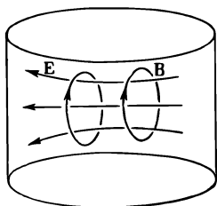
Ф и г. 23.13. Поперечный тип колебаний цилиндрической полости.
