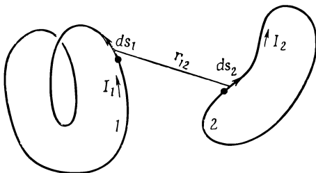
Фиг. 17.9 Любые две катушки обладают взаимной индукцией \mathfrak{M} , пропорциональной интегралу от ds_1 \cdot ds_2 \cdot (1/r_{12}) .
