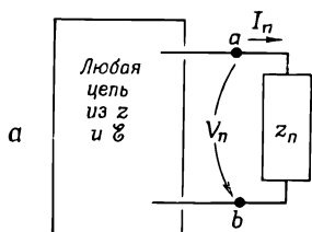
Фиг. 22.16 Любую сеть с двумя выводами можно заменить генератором, последовательно соединенным с импедансом.
