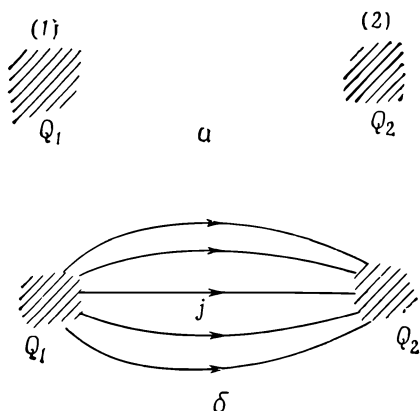
Фиг. 27.1. Два способа описания сохранения заряда.
