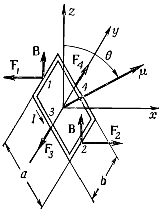
Фиг. 15.1. Прямоугольная петля с током I в однородном поле \mathbf{B} , направленном по оси z . Действующий на нее вращательный момент равен \tau = \mu \times \mathbf{B} , где магнитный момент \mu = Iab
