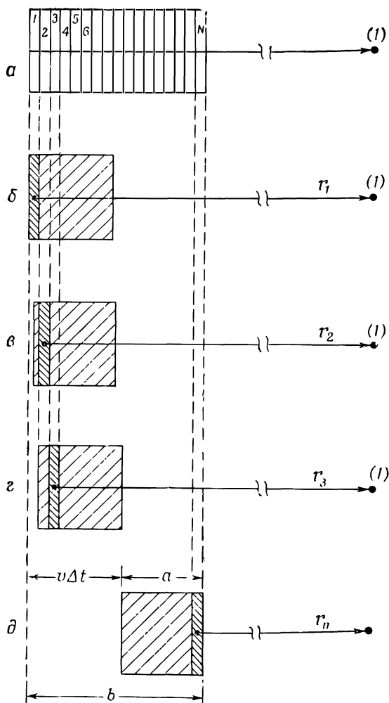
Ф и г. 21.7. Интегрирование \rho(t - r'/c) dV для движущегося заряда.
