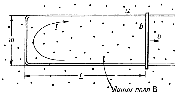
Фиг. 17.1. В рамке наводится э. д. с., если поток меняется за счет изменения площади рамки при перемещении перемычки b .
