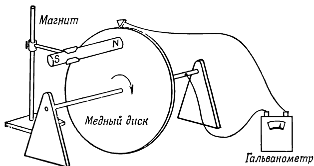
Фиг 17.2. При вращении диска слагаемое \mathbf{v} \times \mathbf{B} порождает э. д. с., но поток сквозь цепь не меняется.
