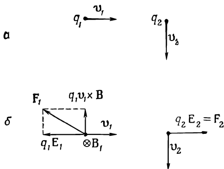
Фиг. 26.6. Силы между двумя движущимися зарядами не всегда равны и противоположны.
