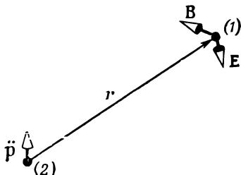
Фиг. 21.4 Поля излучения \mathbf{B} и \mathbf{E} колеблющегося диполя.
