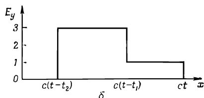
Фиг. 20.3. Если сила источника тока меняется так, как на рисунке (а), то в момент t электрическое поле как функция от x приобретает другой вид (б).
