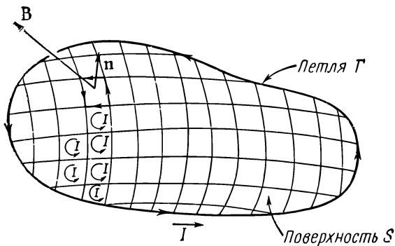
Фиг. 15.4. Энергию большой петли в магнитном поле можно считать суммой энергий маленьких петель.
