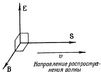
Фиг. 27.2. Векторы \mathbf{E} , \mathbf{B} и \mathbf{S} световой волны.
