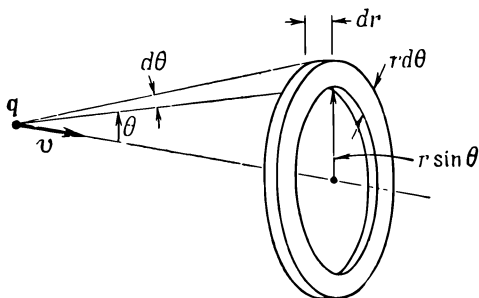
Фиг. 28.2. Элемент объема 2\pi r^2 \sin \theta d\theta dr , используемый при вычислении импульса поля.
