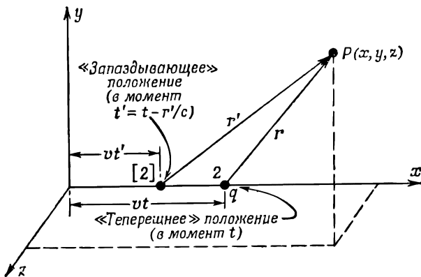
Ф и г. 21.8. Определение потенциала в точке P заряда, движущегося равномерно вдоль оси x .
