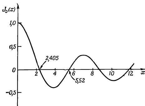
Фиг. 23.6. Функция Бесселя J_0(x) .
