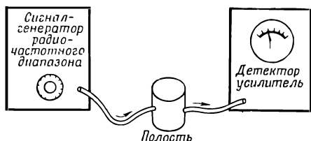
Ф и г. 23.9. Устройство для наблюдения резонанса в полости.
