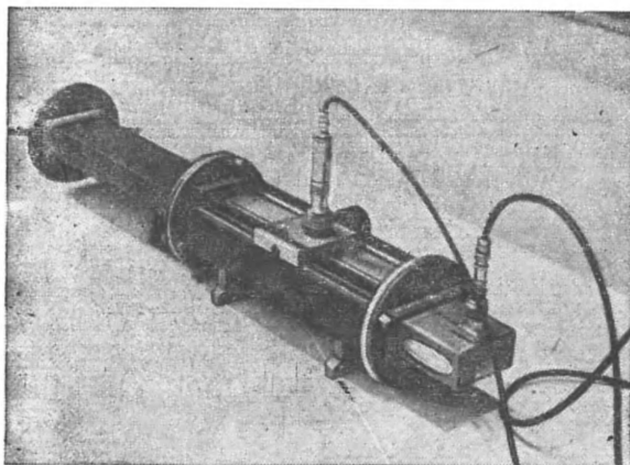
Фиг. 24.9. Секции волновода, соединенные фланцами.
