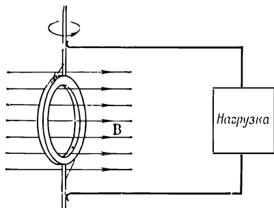
Фиг. 176. Катушка из проволоки, вращающаяся в однородном магнитном поле, — основная идея генератора переменного тока.
