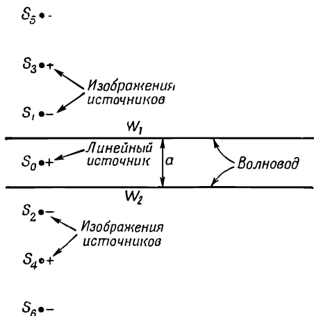
Фиг. 24.15. Линейный источник S_0 между проводящими плоскими стенками W_1 и W_2 . Стенки можно заменить бесконечной последовательностью изображений источников.
