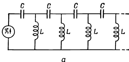
Фиг. 22.23. Высокочастотный фильтр (а) и его фактор распространения как функция от 1/\omega (б).
