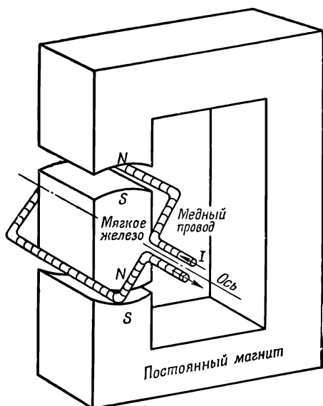
Фиг. 16.1. Схематическое изображение простого электромагнитного мотора.
