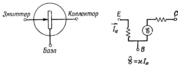
Ф и г. 22.29. Низкочастотная эквивалентная схема транзистора.
