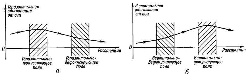
Ф и г. 29.15. Горизонтальная и вертикальная фокусировка парой квадрупольных линз.
