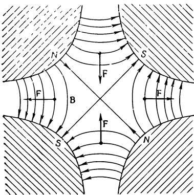
Фиг. 29.13. Горизонтально-фокусирующая квадрупольная линза.
