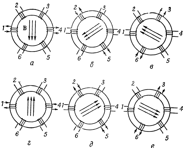
Ф и г. 16.13. Создание вращающегося магнитного поля.
