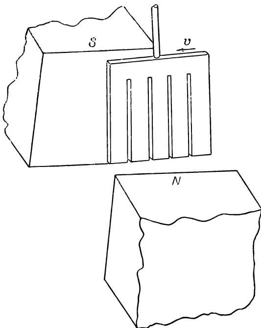
Фиг. 16.12. Эффекты от вихревых токов сильно снижаются, если в пластинке прорезать щели.
