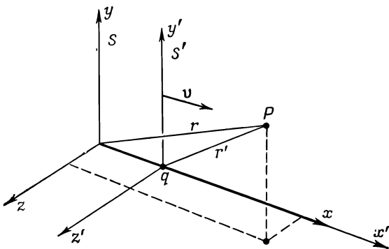
Фиг. 25.2. Система отсчета S' движется со скоростью v (в направлении оси x ) по отношению к системе S .
