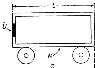
Фиг. 27.7. Порция энергии U , движаясь со скоростью c , несет импульс, равный U/c .
