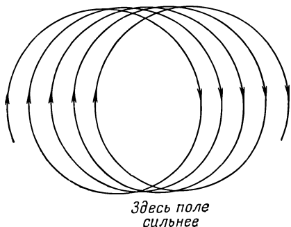
Фиг. 29.10. Движение частицы в слабо неоднородном поле.
