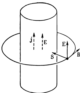
Фиг. 27.5. Вектор Пойнтинга \mathbf{S} вблизи провода с током.
