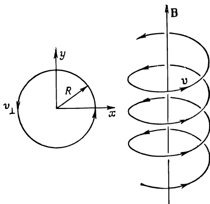
Фиг. 29.1. Движение частицы в однородном магнитном поле.
