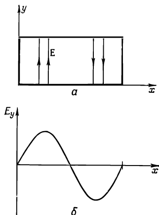
Ф и г. 24.14. Еще одна возможная зависимость E_y от x .
