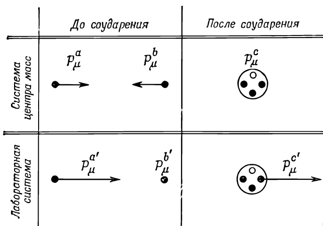
Фиг. 25.1. Реакция p + \bar{p} \rightarrow 3p + \bar{p} в лабораторной системе и системе ц. м.
