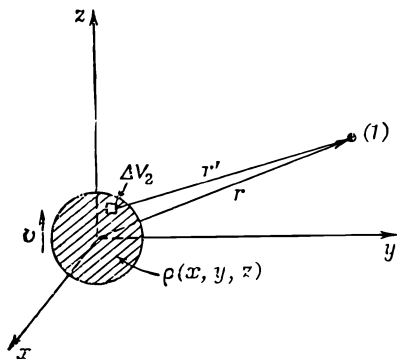
Фиг. 21.2. Потенциалы в точке (I) даются интегралами от плотности заряда \rho .
