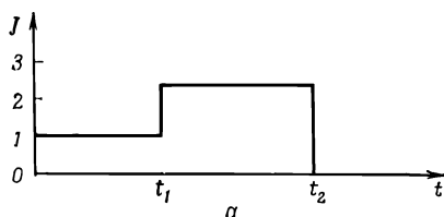
Фиг. 20.3. Если сила источника тока меняется так, как на рисунке (а), то в момент t электрическое поле как функция от x приобретает другой вид (б).
