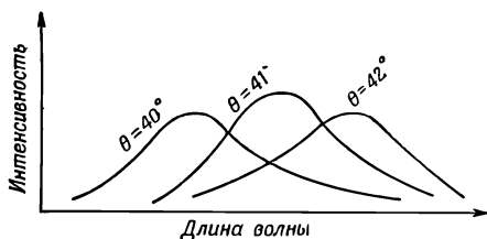
Фиг. 20.5. Зависимость интенсивности электромагнитных волн от длины волны под тремя углами (отсчитываемыми от направления, противоположного направлению на Солнце). Доступно наблюдению лишь в определенных метеорологических условиях
