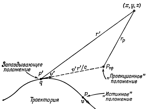
Ф и г. 26.2. Движение заряда по произвольной траектории.
