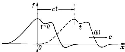
Фиг. 20.4. Функция f(x - ct) представляет неизменный «коптур», движущийся в направлении возрастания x со скоростью c .
