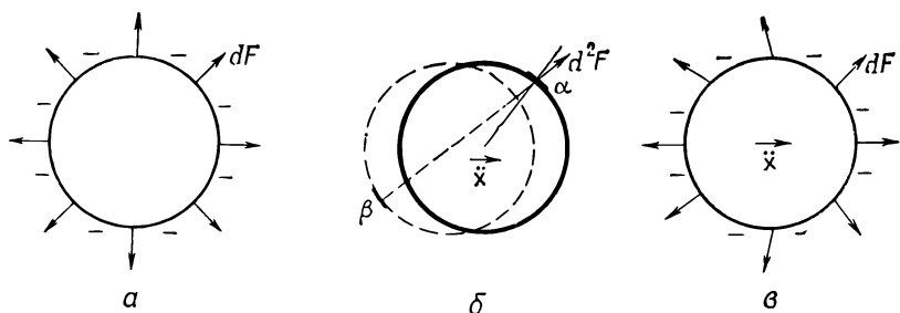
Фиг. 28.3. Сила действия ускоряющегося электрона благодаря запаздыванию не равна нулю.
