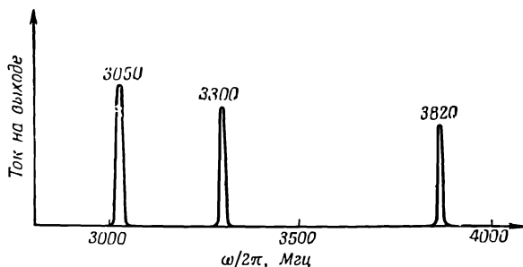
Фиг. 23.11. Наблюдаемые резонансные частоты цилиндрической полости.
