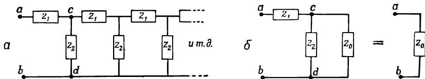
Фиг. 22.19. Эффективный импеданс бесконечной лестницы.
