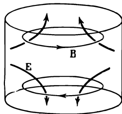
Ф и г. 23.14. Еще один тип колебаний цилиндрической полости.
