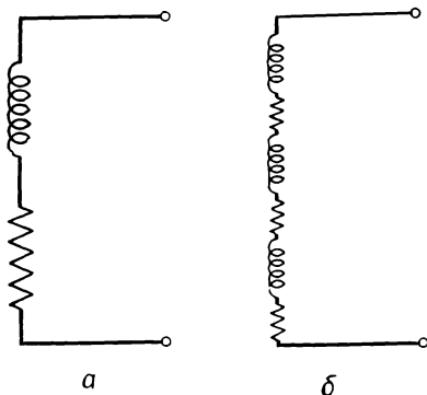
Ф и г. 23.2. Эквивалентная схема реальной индуктивности на низких частотах.
