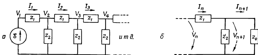
Фиг. 22.21. Нахождение фактора распространения лестницы.
